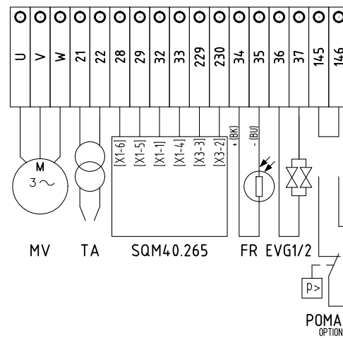
QG - MC MORSETTIERA ALIMENTAZIONE SUPPLY TERMINAL BOARD
