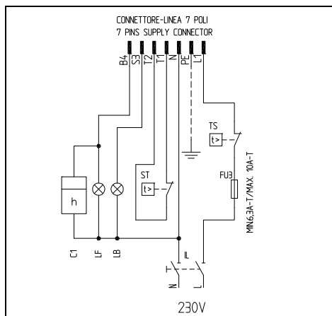
Fig. 7 - Connettore 7 poli
