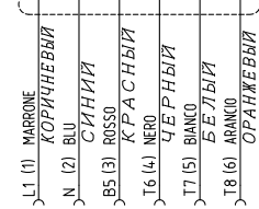
CONN. SONDE
