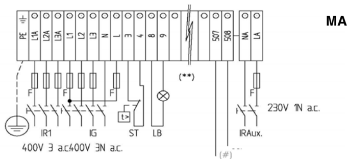
Fig. 2 - Bruciatori modulanti
