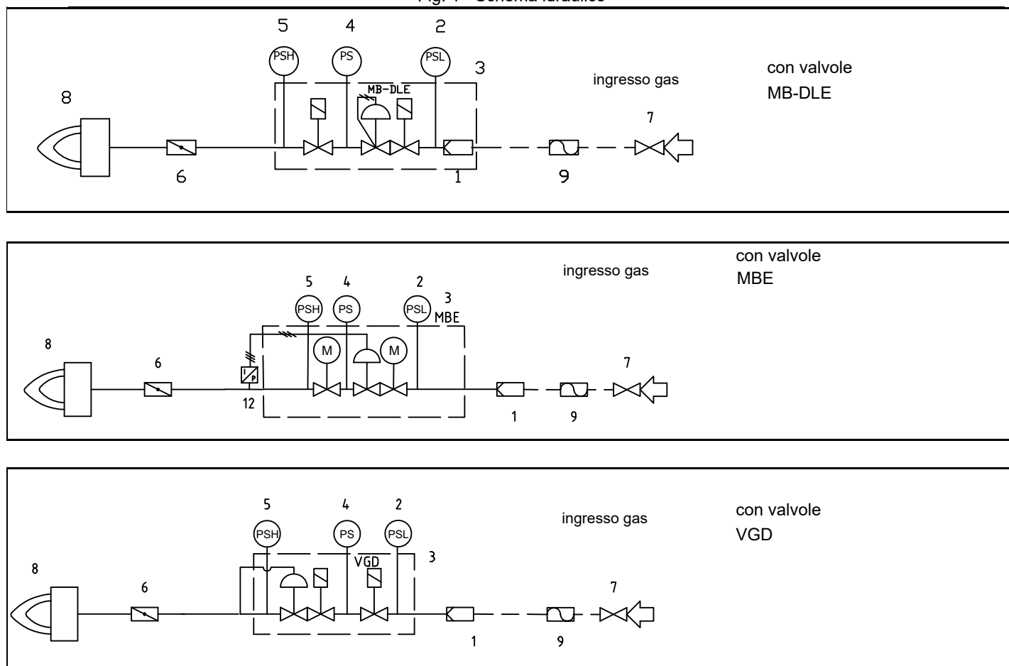
Fig. 1 - Schema idraulico
