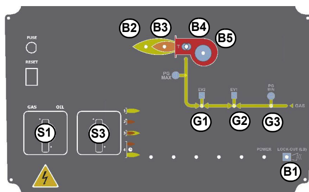
Pannello frontale quadro elettrico bruciatore
