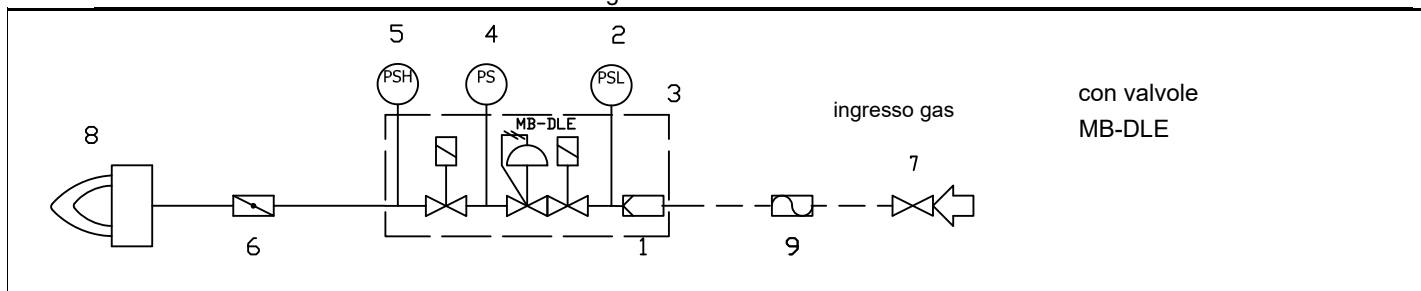
Fig. 1 - Schema idraulico
