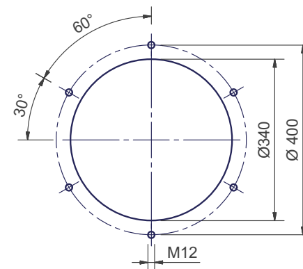
Foratura caldaia consigliata
