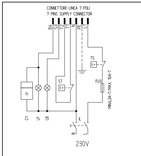
Fig. 34 - 7-polige Steckverbindung
