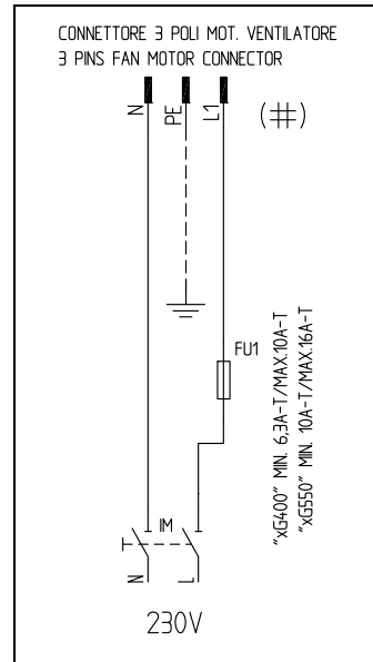
Fig. 35 - 3-polige Steckverbindung Elektromotor NG/LG/NGX400
