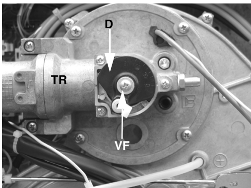
Fig. 21: Standard-Stellung
