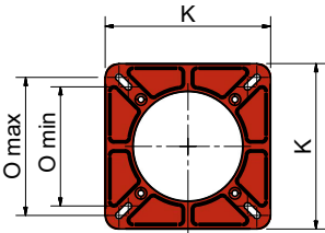
Flangia bruciatore
