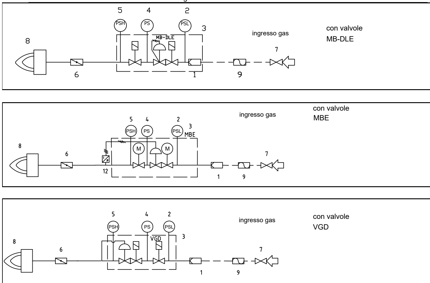
Fig. 2 - Schema idraulico
