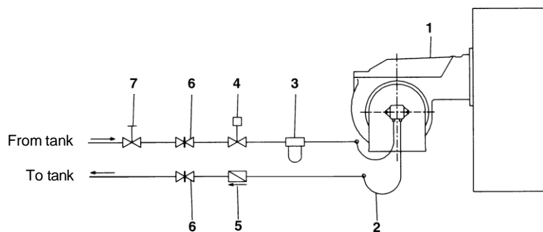
Fig. 21 - Zwei-Rohr-System
