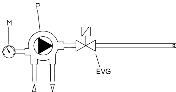
Abb. 30 - Einstufige Brenner
