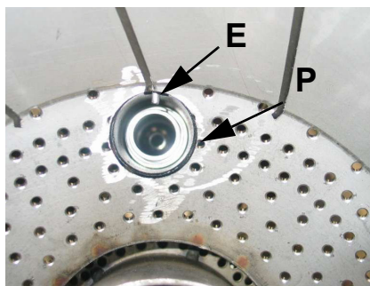
- Particolare del diffusore con pilota (P) e elettrodo di accensione (E)
