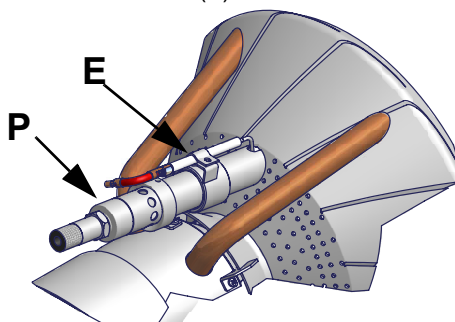
- Particolare del diffusore con pilota (P) e elettrodo di accensione (E)
