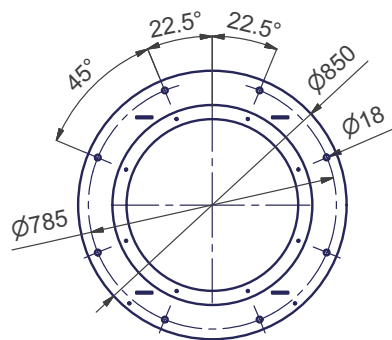
РЕКОМЕНДУЕМАЯ АМБРАЗУРА КОТЛА
