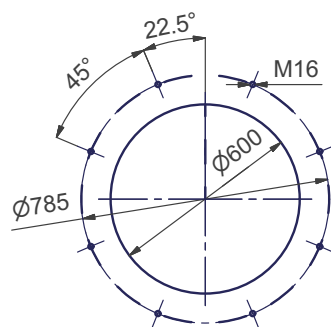
ФЛАНЕЦ ГОРЕЛКИ
