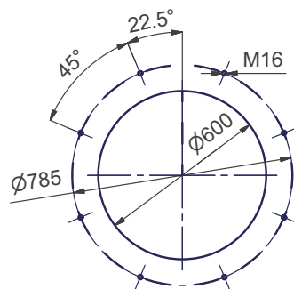
ФЛАНЕЦ ГОРЕЛКИ
