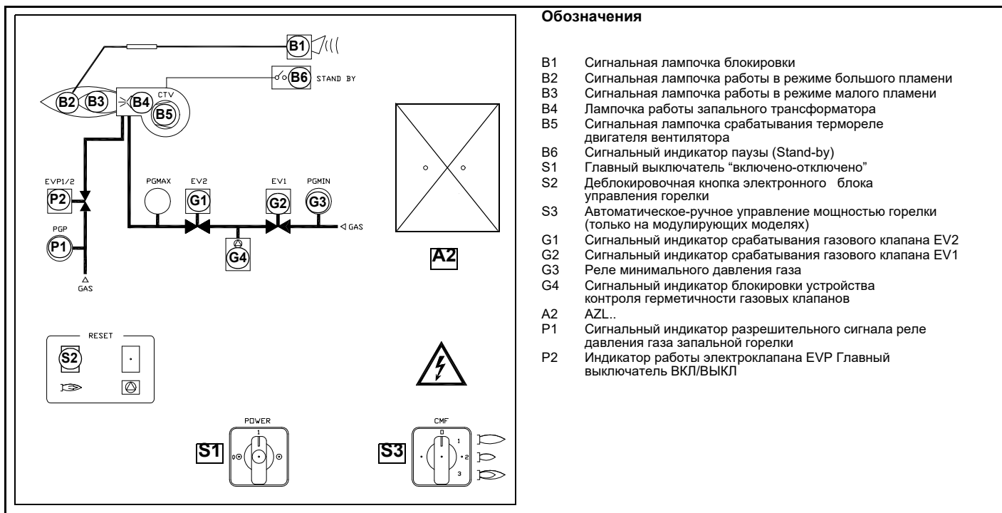
Рис. 1 - Лицевая панель электрощита
