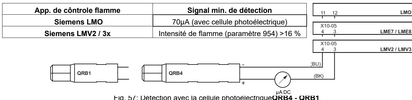
Fig. 57: Détection avec la cellule photoélectrique QRB4 - QRB1
