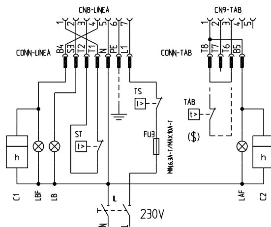
Fig. 20: Brûleurs à deux allures
