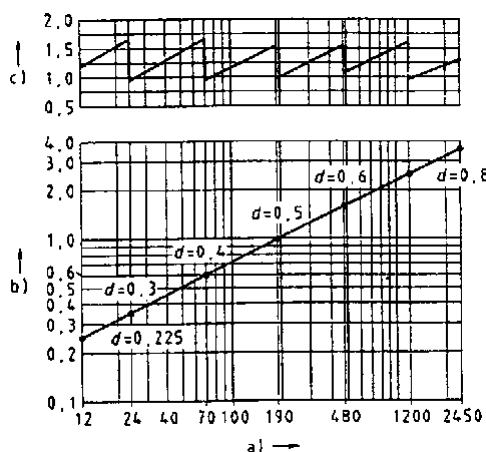
Fig.3: Charge thermique, diamètre et longueur du foyer d'essai en fonction de la puissance brûlée Q
