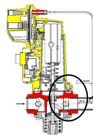
Siemens VGD... con SKPx Пример газовой рампы
