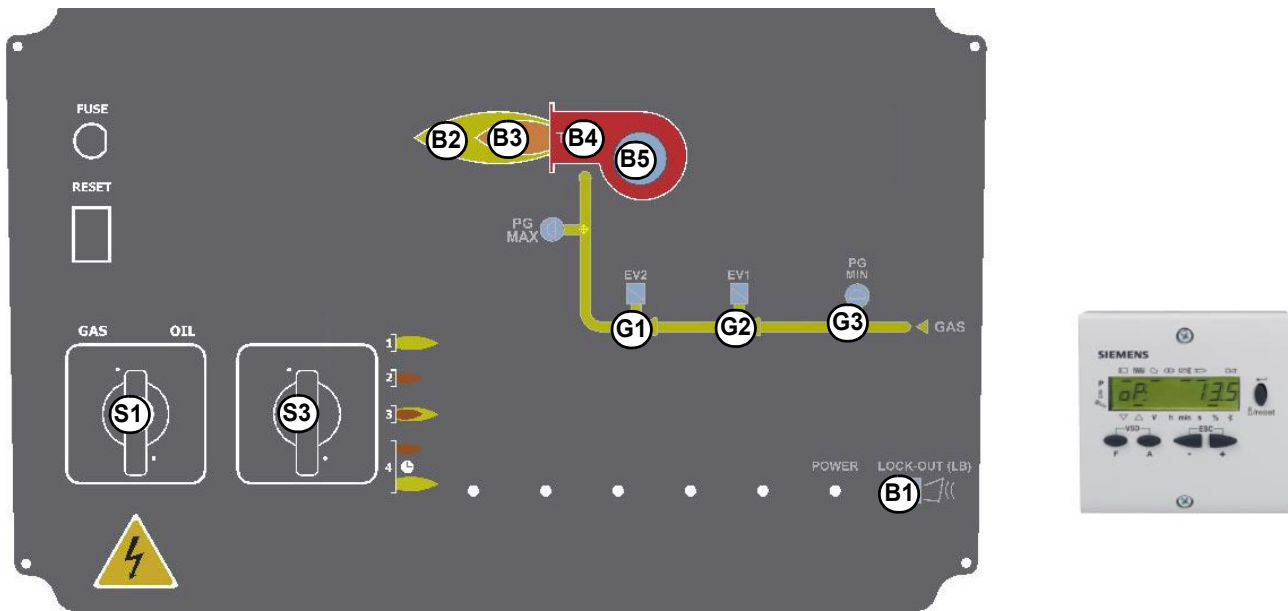
Fig. 4 Panel frontal cuadro eléctrico
