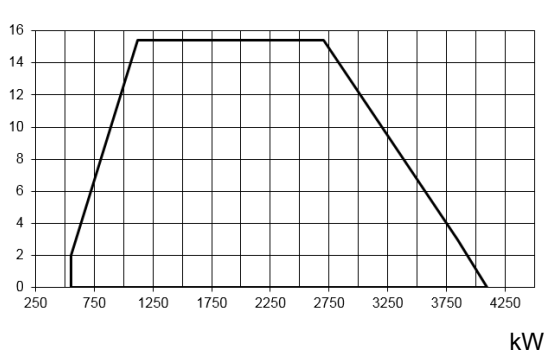
KP93 L-
