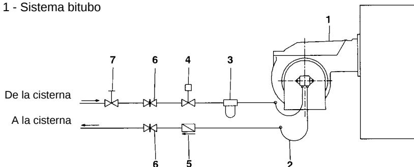
Fig. 1 - Sistema bitubo
