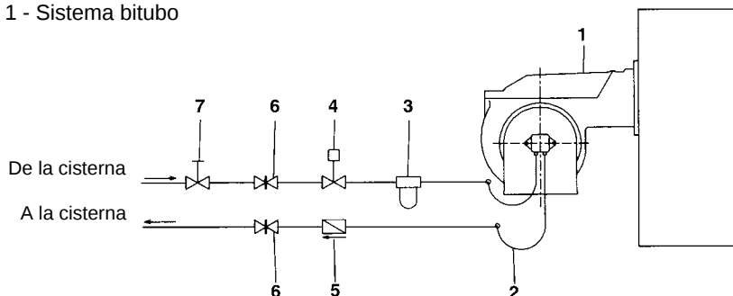
Fig. 1 - Sistema bitubo
