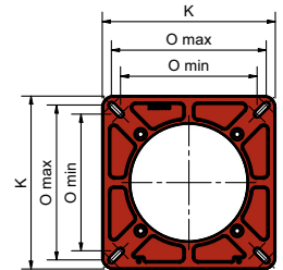
flangia bruciatore
