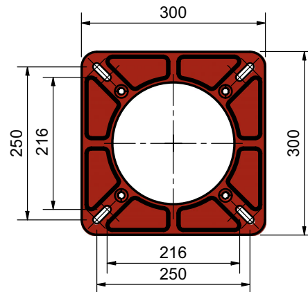
Flangia bruciatore
