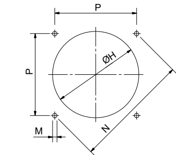
Схема сверления плиты котла
