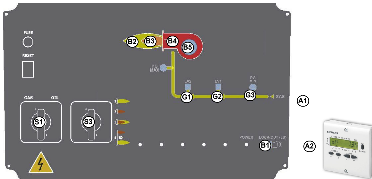
Рис. 1: передняя панель электрощита горелки
