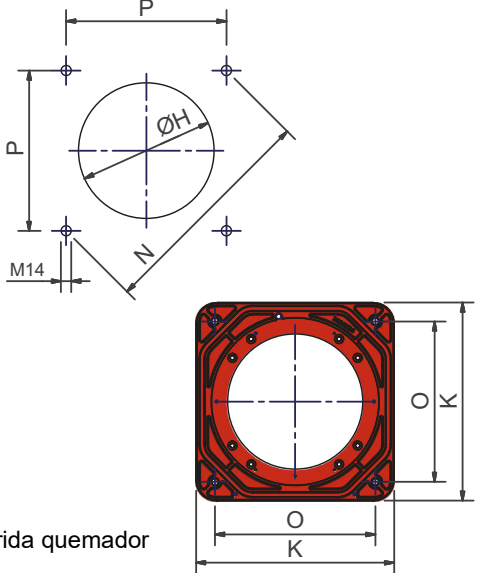
Plantilla de perforación recomendada de la placa de la caldera.
