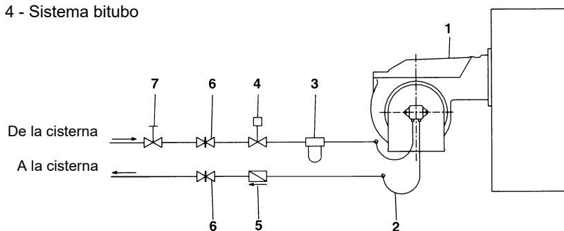
Fig. 4 - Sistema bitubo
