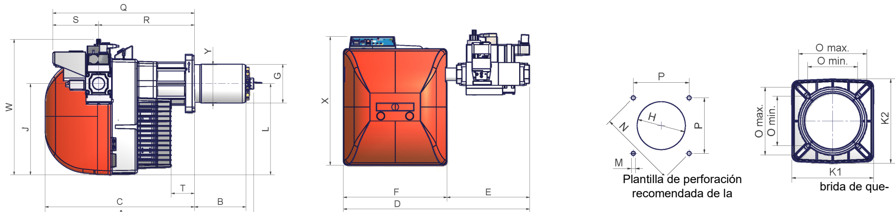
Perforación caldera recomendada y brida quemador
