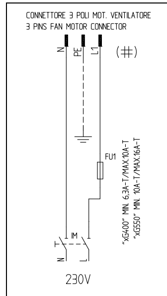
Fig. 19 - Conector 3-polos por el motor eléctrico de NG/LG/NGX400
