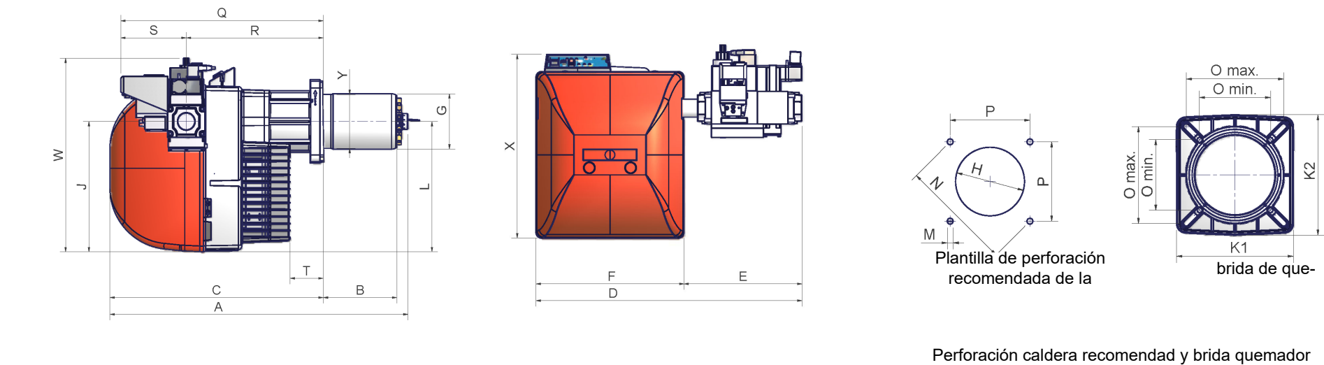
Perforación caldera recomendada y brida quemador
