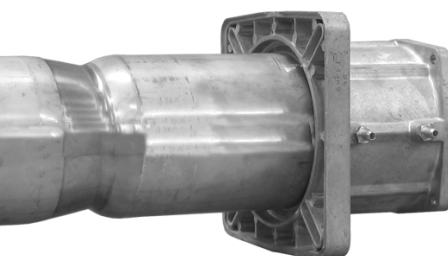
Fig. 5 - Tobera en versión larga
