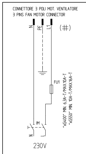
Fig. 21 Conector 3-polos por motor eléctrico NG/LG/NGX400
