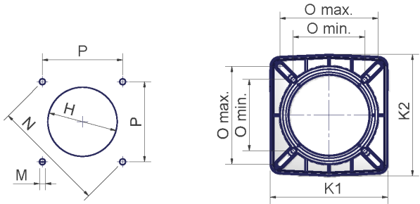
brida de quemador
