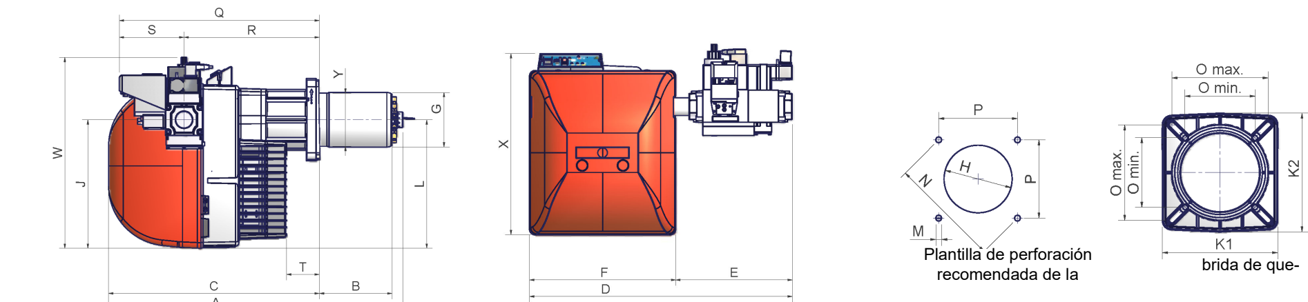
Perforación caldera recomendada y brida quemador
