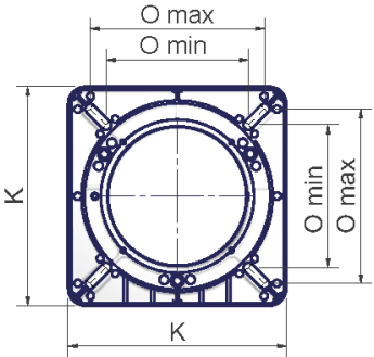
bride brûleur
