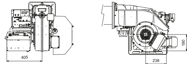
Dimensiones con Inverter
