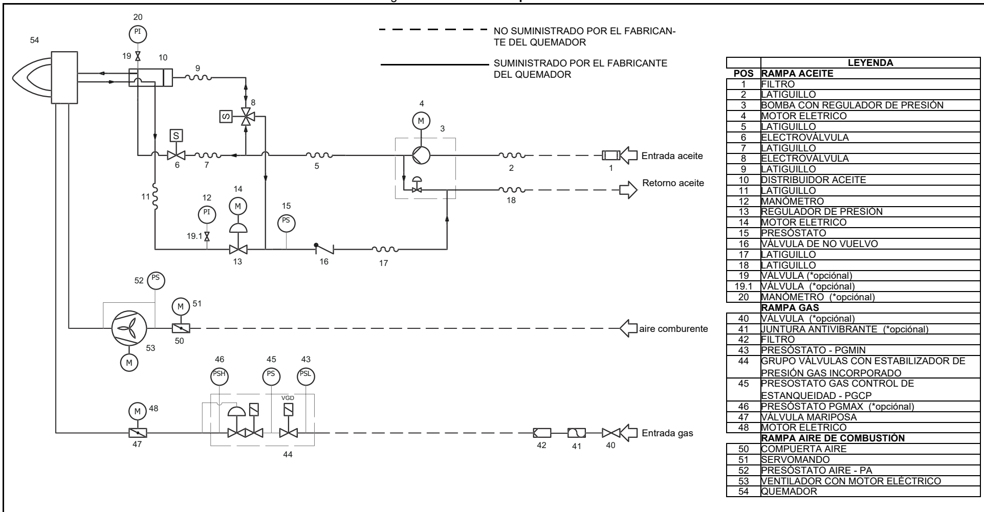
Fig. 2 - 3I2MG-23 v0 Esquema hidráulico
