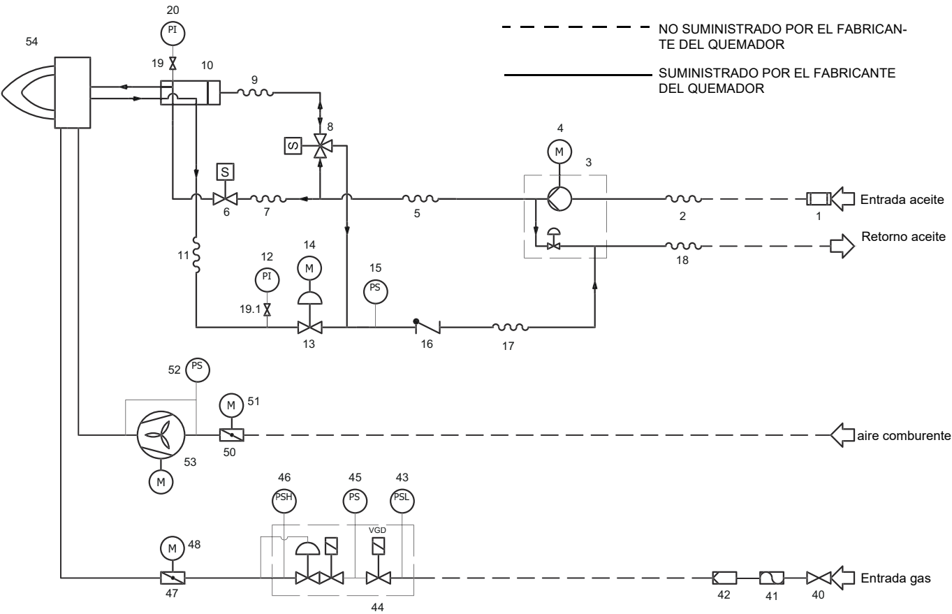
Fig. 2 - 3I2MG-23 v0 Esquema hidráulico
