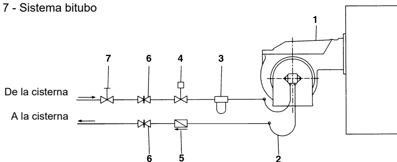
Fig. 7 - Sistema bitubo
