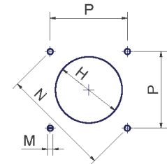
Gabarit de perçage plaque chaudière
