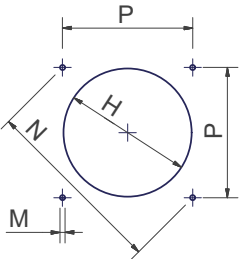
Gabarit de perçage plaque chau- dière
