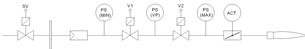
Fig. 10. Accensione diretta (rampa gas)
