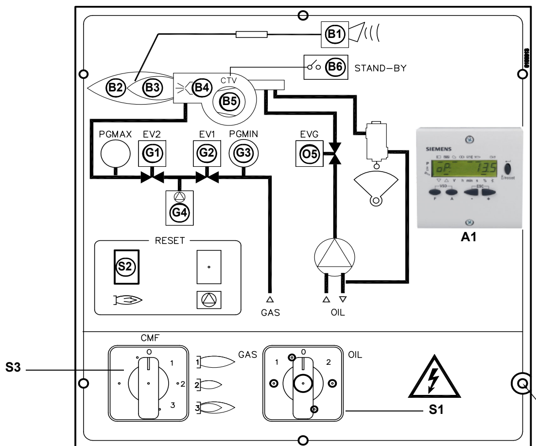
Fig. 1 - Panelo cuadro electrico
