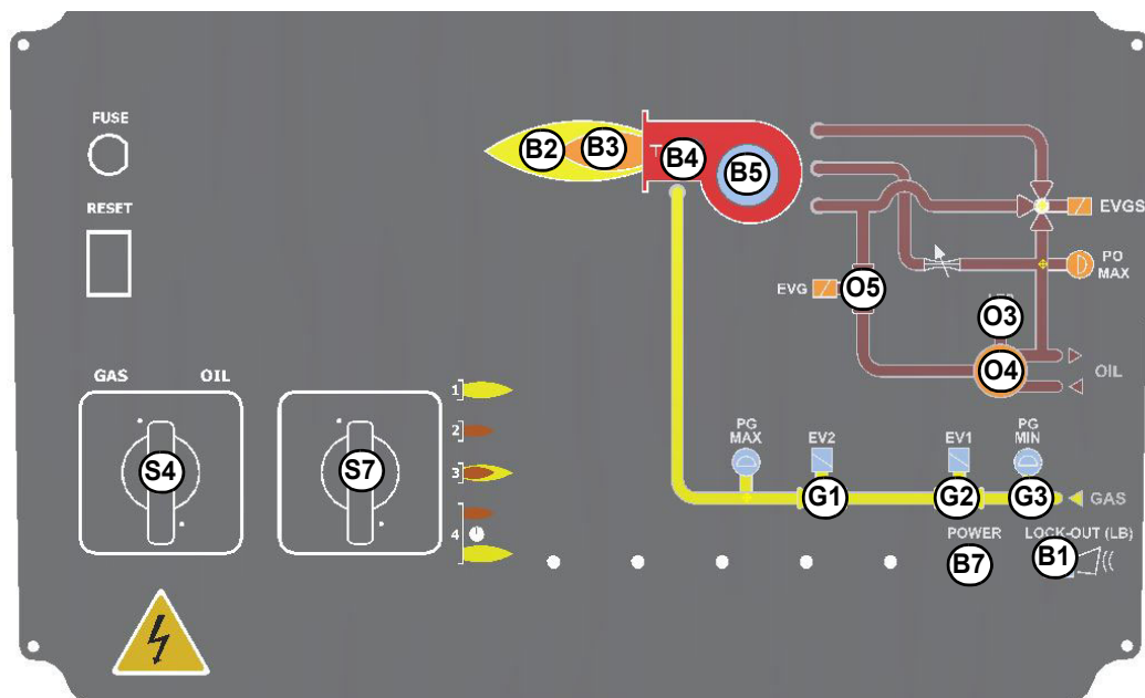
Fig. 7 - Pannello frontale quadro elettrico bruciatore
