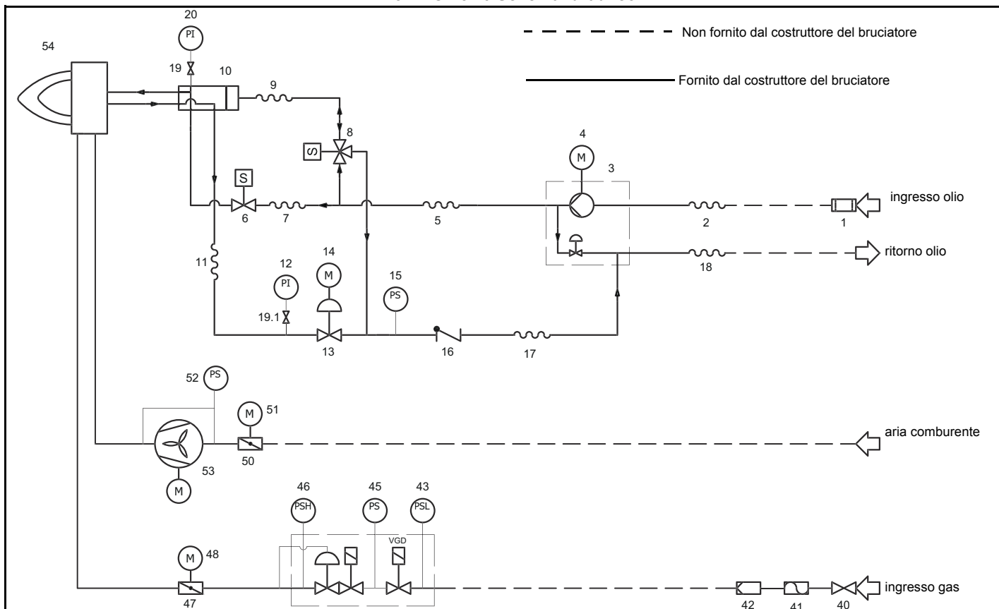
Fig. 2 - 3I2MG-23 v0 Schema idraulico
