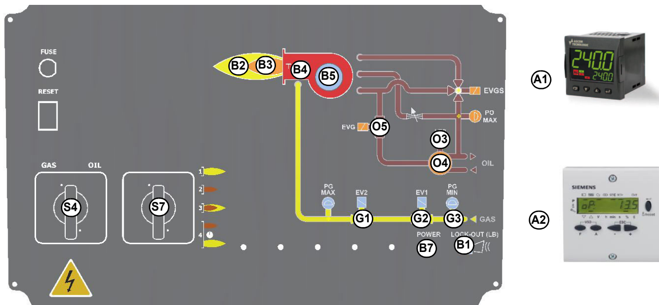
Fig. 7 - Panel frontal quemadores
