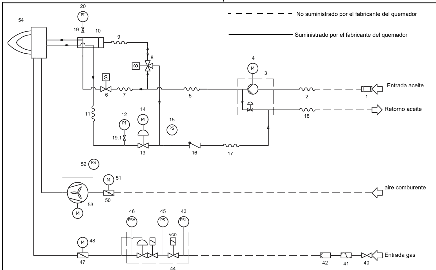
Fig. 2 - 3I2MG-23 v0 Esquema hidráulico
