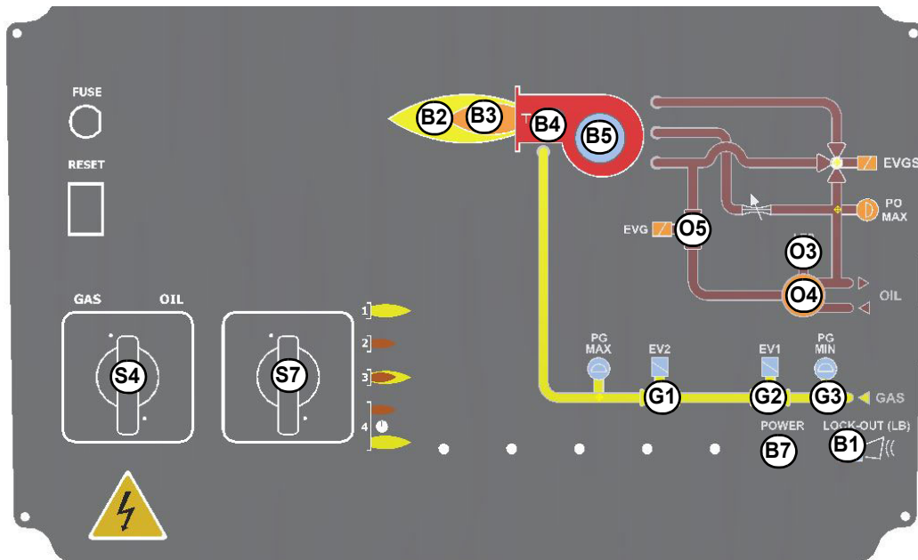
Fig. 7 - Panel frontal quemadores
