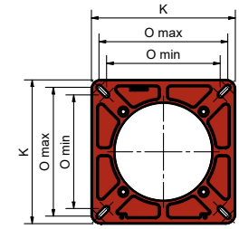
фланец горелки
