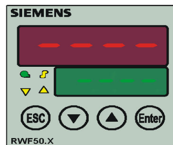
Рис. 42 - RFW50 : МОДУЛИРУЮЩИЙ РЕГУЛЯТОР
