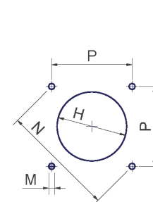
Рекомендуемая амбразура котла
