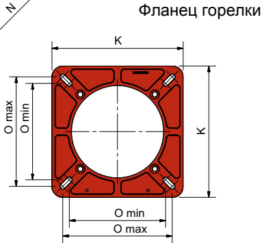
Фланец горелки
