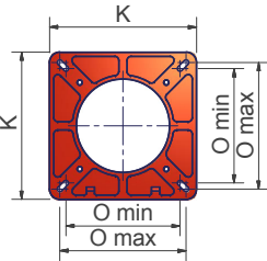
Фланец горелки
