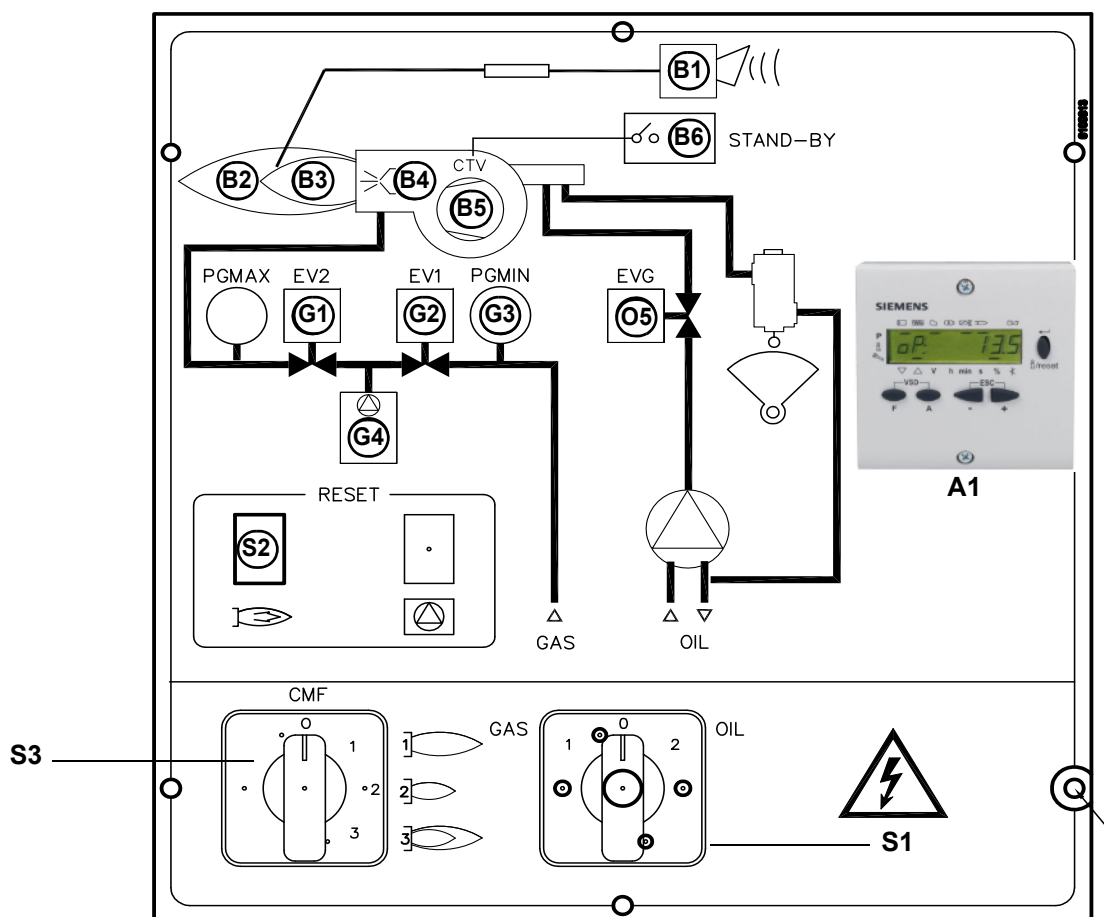
Fig. 1 - Panoelo cuadro electrico
