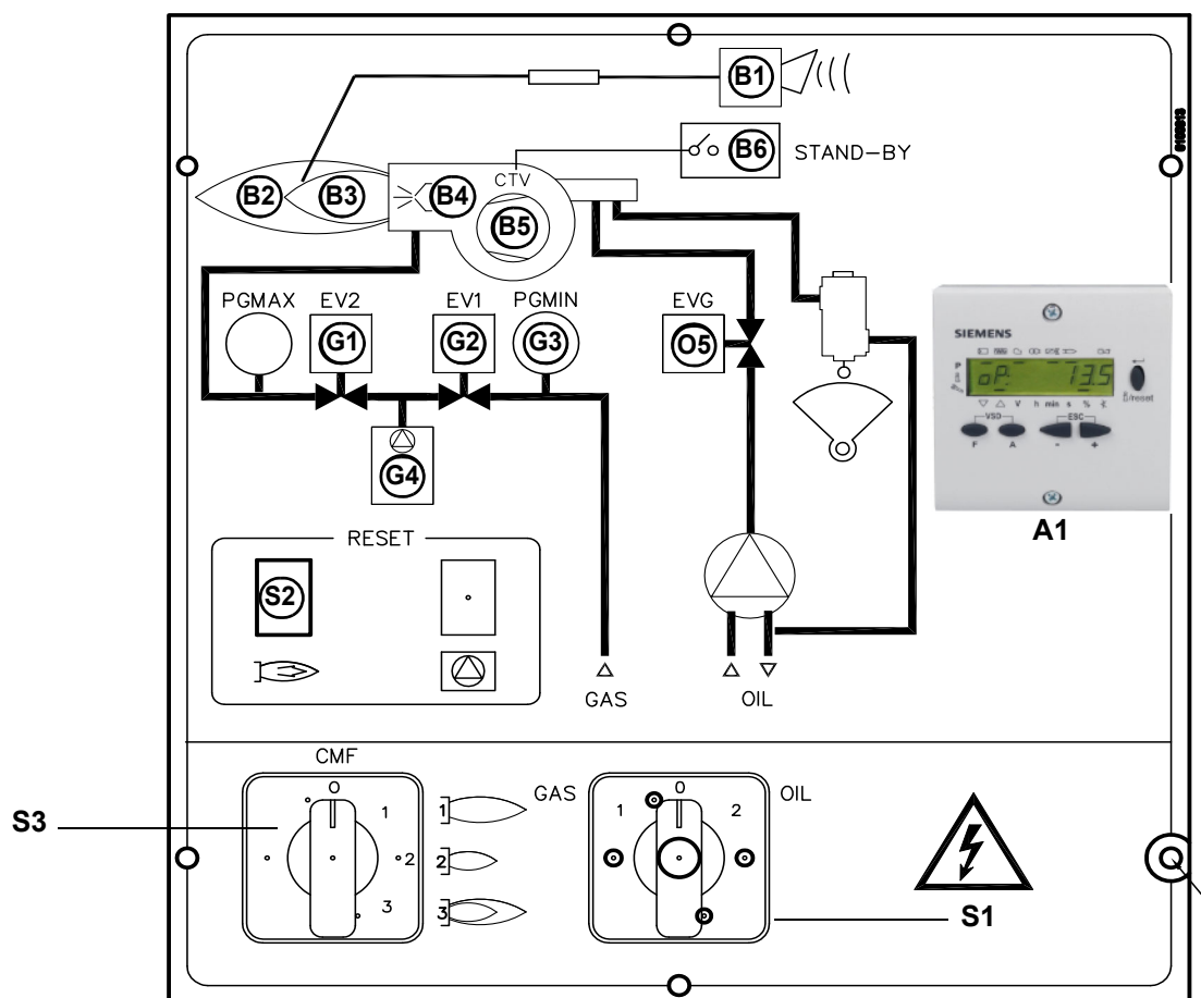
Fig. 1 - Pannelo cuadro electrico
