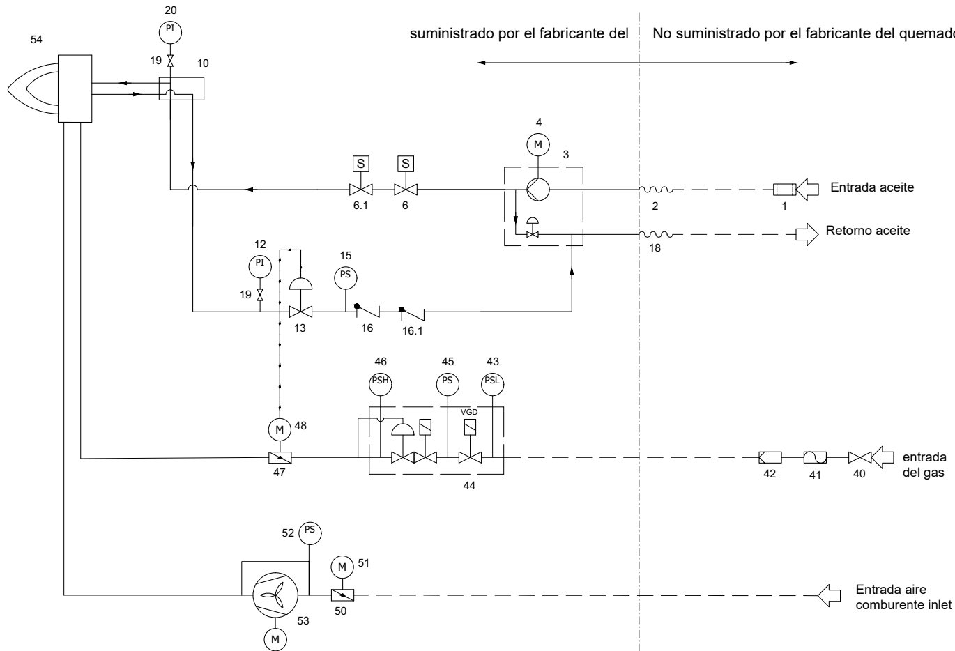
Fig. 3Esquema hidráulico 3I2MG78
